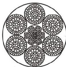
8X103FSNS+IWR
