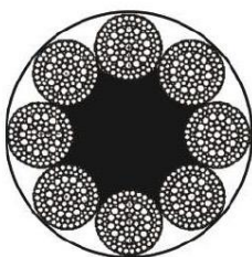
8X103FSNS+FC
