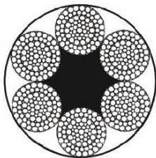
6X84WSNS+FC
