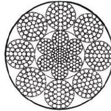
8x37+IWR
