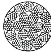
18x19W+IWS
