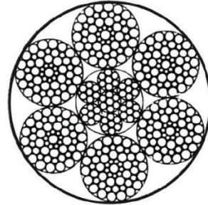
6x55SWS+IWR
