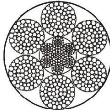
6X65FNS+IWR
