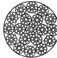
18x19S+IWS
