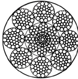
8x36WS+IWR
