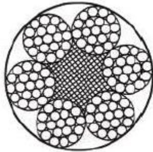
6x19+FC
