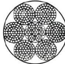
6x61+IWR
