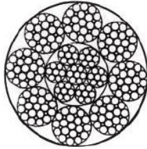
8x25Fi+IWR
