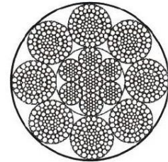
8X80WSNS+IWR
