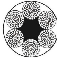
6X80WSNS+FC
