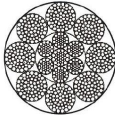
8X65FNS+IWR
