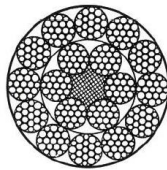
18x19W+FC
