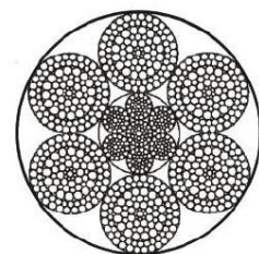
8X109SWSNS+IWR
