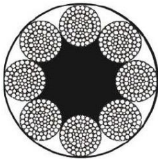
8X84WSNS+FC
