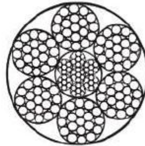
6x19+IWR
