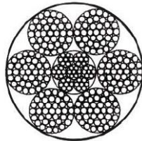
6x37+IWR
