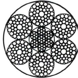
6x41WS+IWR
