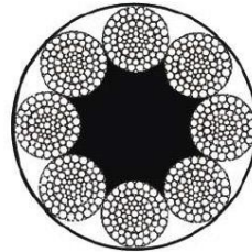
8X80WSNS+FC
