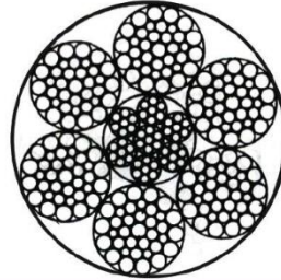
6x36WS+IWR
