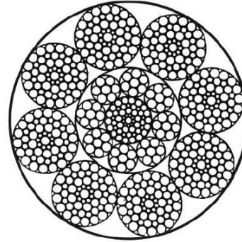
8x55SWS+IWR
