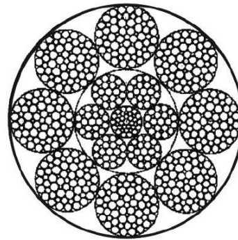
8x61FWS+IWR
