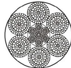
6X109SWSNS+IWR
