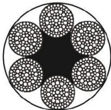
6X103FSNS+FC
