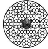
18x7+FC
