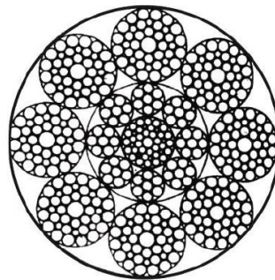
8x41WS+IWR
