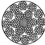
18x19+FC
