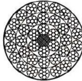
36x7+FC
