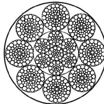
8x64SFS+IWR
