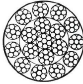
17x7+IWS
