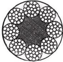
8x25Fi+FC
