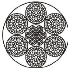
6X103FSNS+IWR
