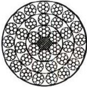
34x7+FC
