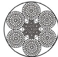
6X111SWSNS+IWR
