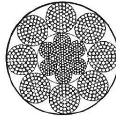
8x61+IWR
