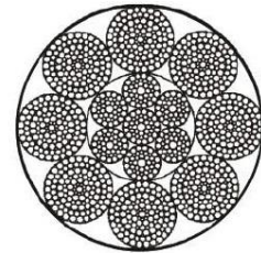
8X111SWSNS+IWR
