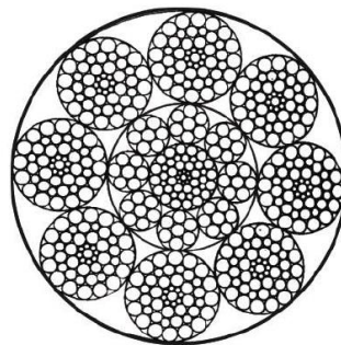
8x49SWS+IWR
