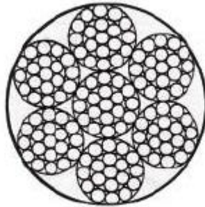
6x19+IWS
