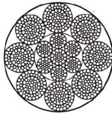
8X84WSNS+IWR
