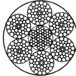
6x49SWS+IWR
