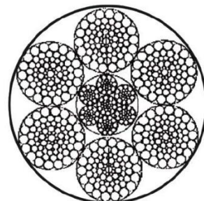
6x64SFS+IWR
