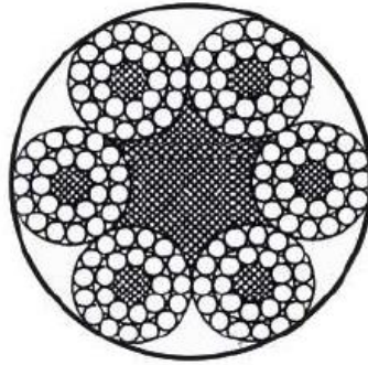
6x24+7FC
