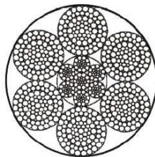
6X84WSNS+IWR
