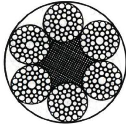
6x41WS+FC
