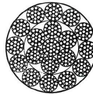
18x19+IWS
