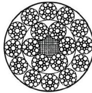
18x19S+FC
