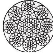
8x31WS+IWR
