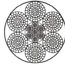
6X80WSNS+IWR
