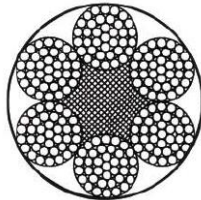
6x37+FC
