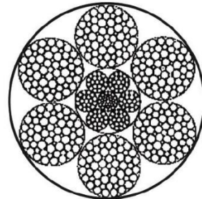
6x61FWS+IWR
